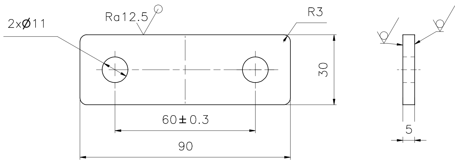
Item no.5 ( 1 : 1 )
