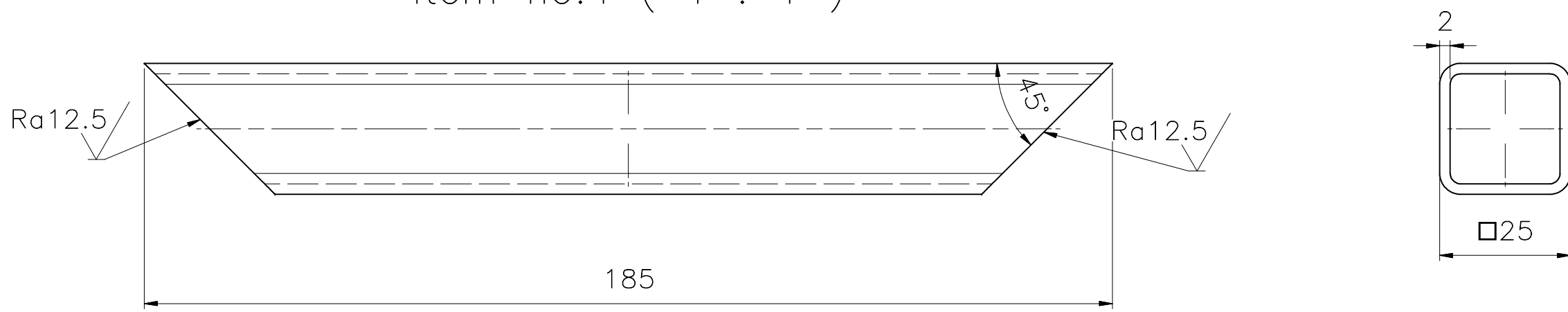
Item no.4 ( 1 : 1 )
