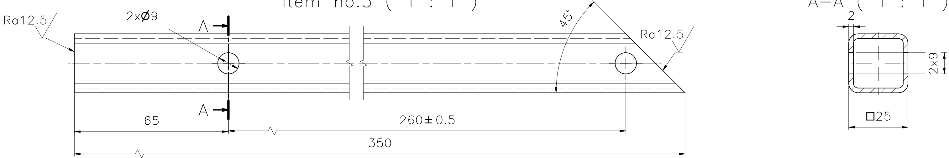
Item no.3 ( 1 : 1 )
