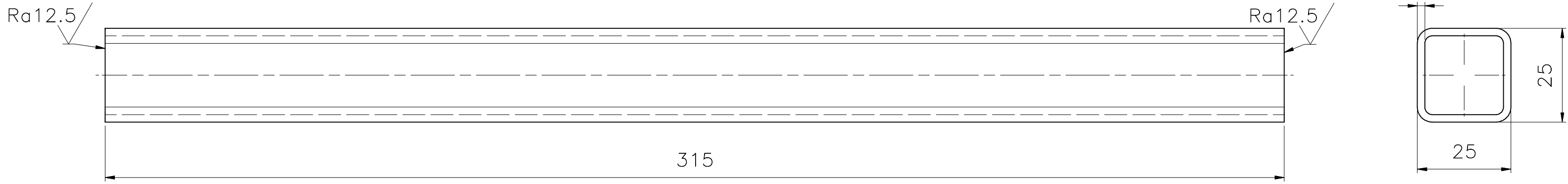
Item no.2 ( 1 : 1 )
