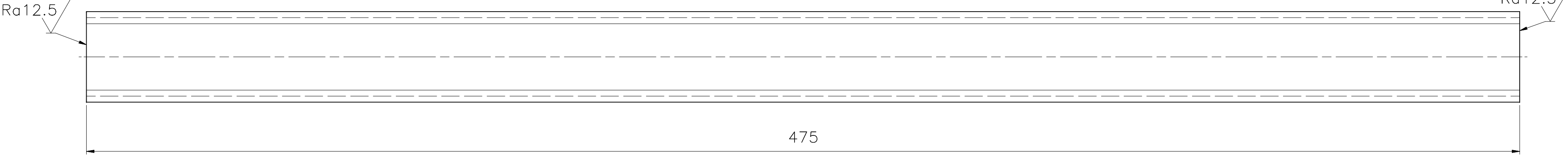
Item no.1 ( 1 : 1 )
